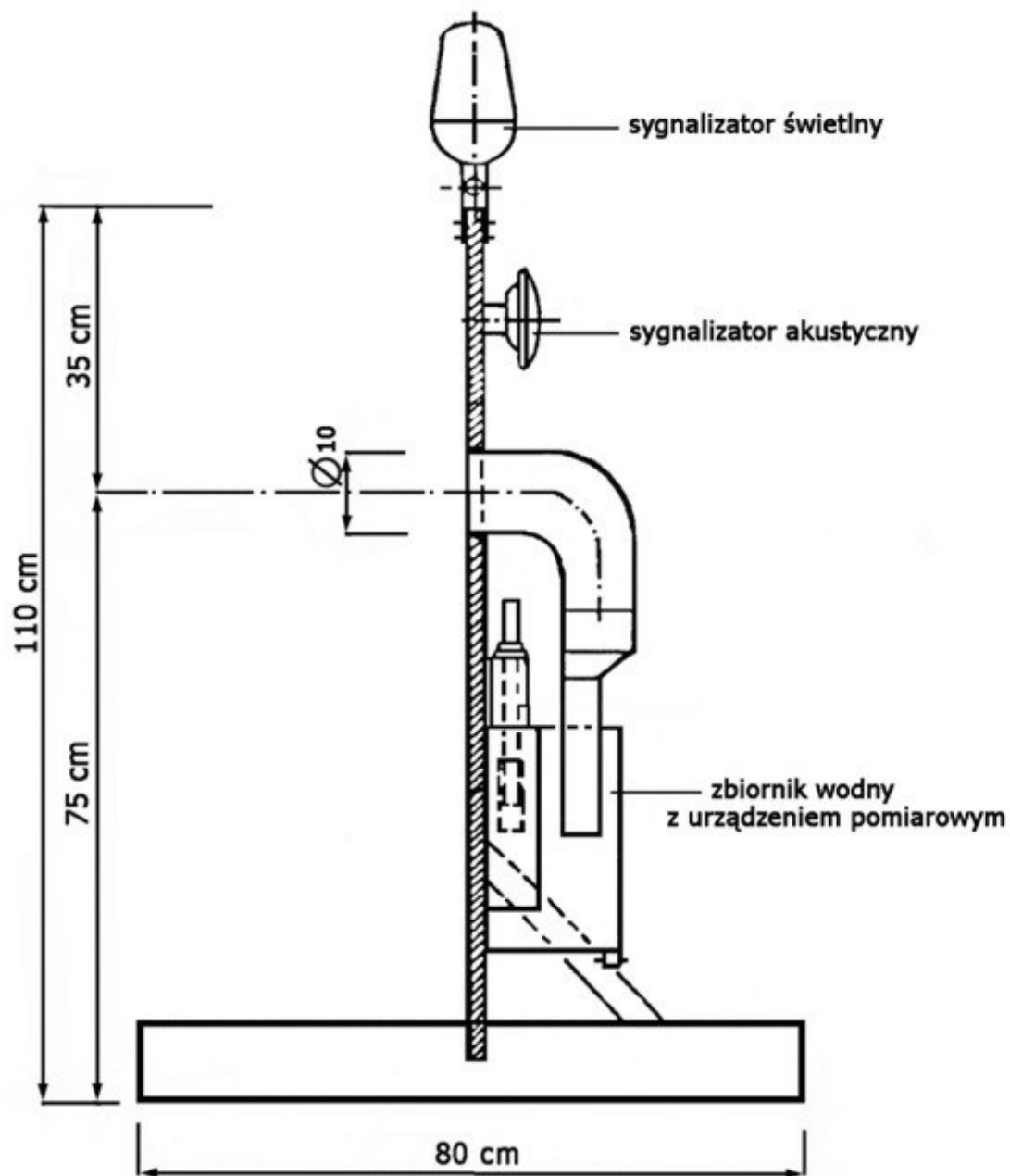
Rys. 6. Tarcza nalewowa
