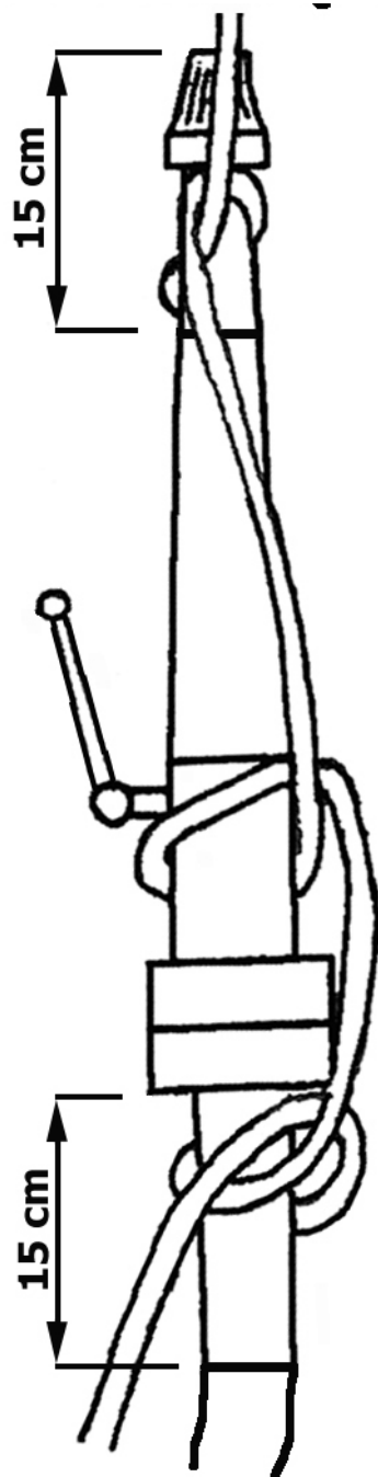
Rys. 10. Cała pętla na prądownicy z półpętłą
